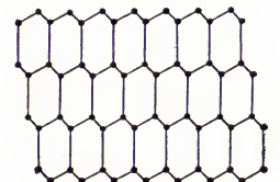
Правильная система точек на плоскости.
